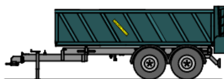
AgroMax Plus TA-180 Tsz / AgroMax Plus TA-240 Tsz 6,2x2,1x1,5 m / 7,2x2,1x1,5 m
